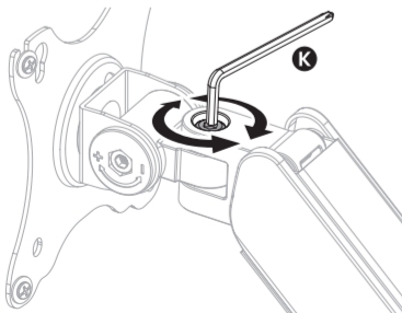
2. Wenn die Einstellung schwierig ist, ziehen Sie die angegebene Schraube je nach Bedarf fest oder lockern Sie sie.
